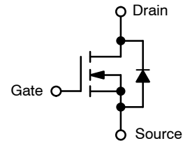
MMBF170 SOT-23 CASE 318-08
